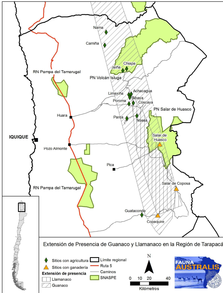
Figura 8. Sobre-posición de extensión de la presencia de guanacos y llamanacos
